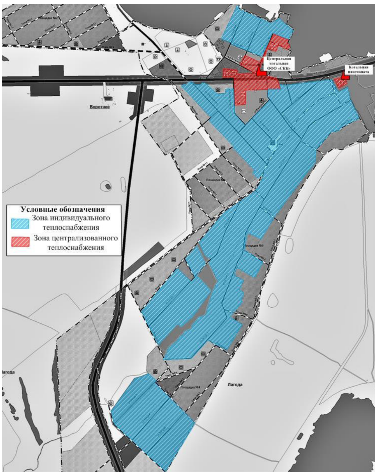
Рис. № 2 - Зоны действия Центральной котельной, Котельной пансионата и индивидуальных источников тепловой энергии на территориях села Воротнее и поселка Лагода
