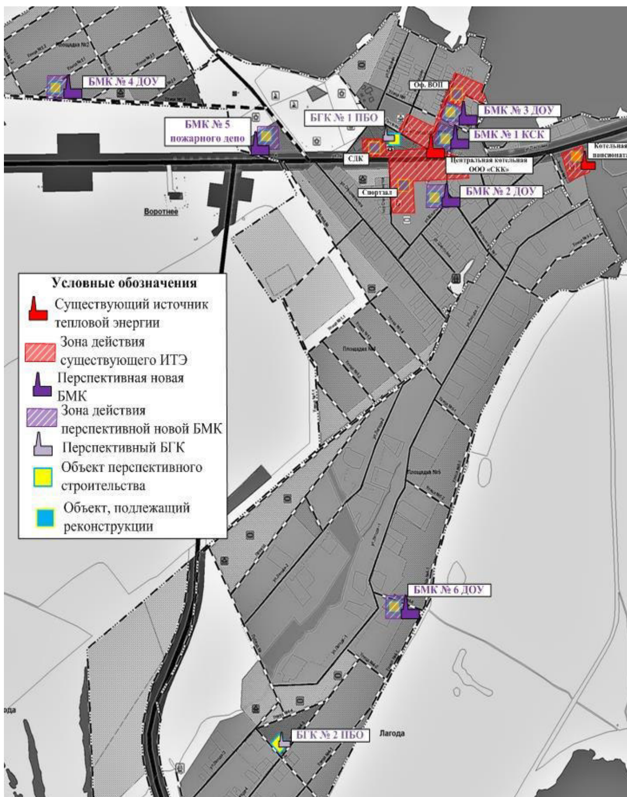
Рис. № 14 – Перспективные зоны теплоснабжения существующих котельных и перспективных источников т. э. на территориях села Воротное и поселка Лагода
